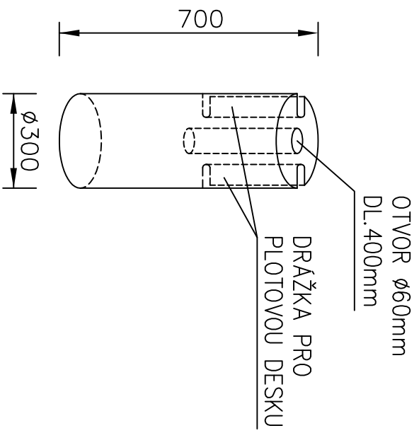
PATKA PLOTOVÁ 700x300
