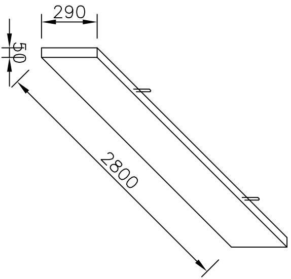
DESKA PLOTOVÁ 2800x290x50
